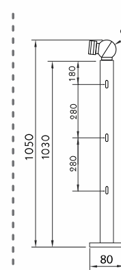
05 POSTE S/ PESC. BARRA EXT. 16MM
