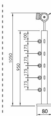
02 POSTE BARRA EXT. CANTO
