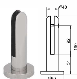
C130 - Pinça redonda vidro 10/12/16mm
