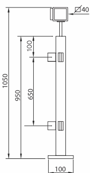
POSTE QUADRADO CANTO VIDRO
