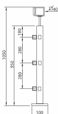
POSTE QUADRADO BARRA EXTERNA CANTO 15mm
