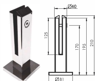
C139 - Pinça Eco vidro 10mm
