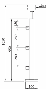
POSTE QUADRADO BARRA EXTERNA 15mm
