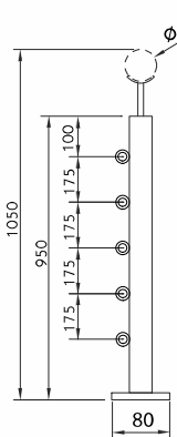
01 POSTE BARRA EXT. 12.7mm
