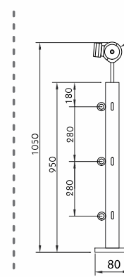
04 POSTE BARRA EXT. CANTO
