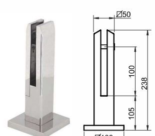
C131 - Pinça quadrada vidro 10/12/16mm
