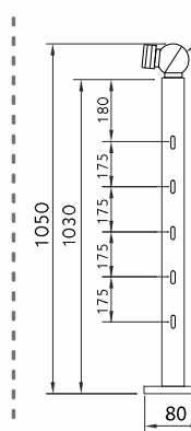
03 POSTE S/ PESC. BARRA EXT. 12.7MM
