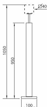
POSTE QUADRADO LISO
